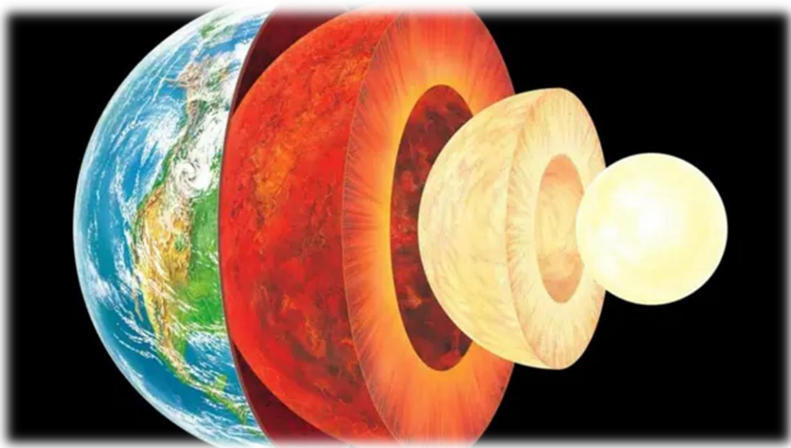
Figure 1. L'image de la Terre en profil (de la surface en profondeur)
