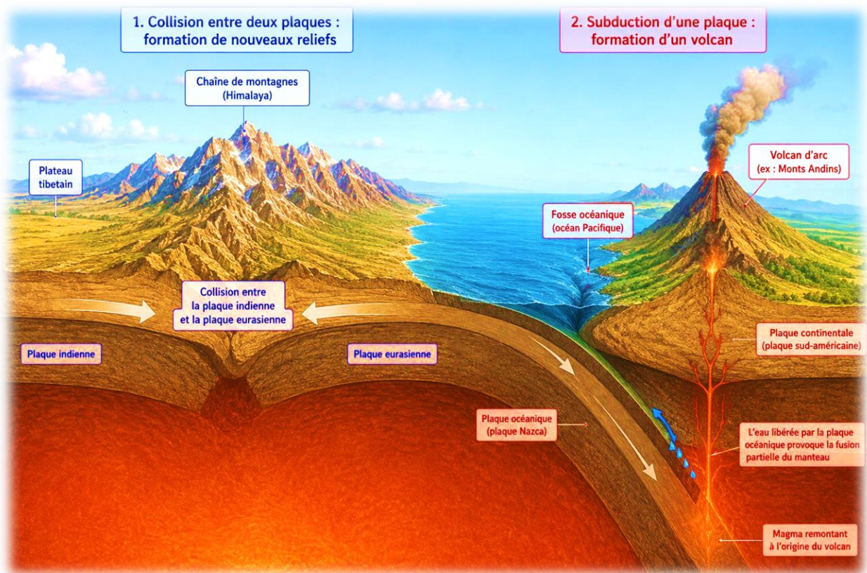
Figure 2. Exemples d'une collision et d'une subduction des plaques tectoniques
